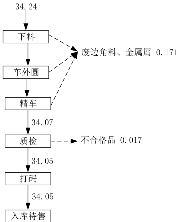
图 2 物料平衡图
