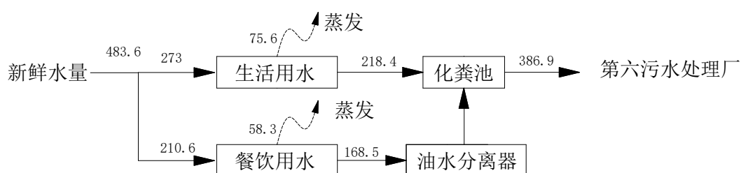
图2 项目水平衡图 (单位: m 3 /a)
