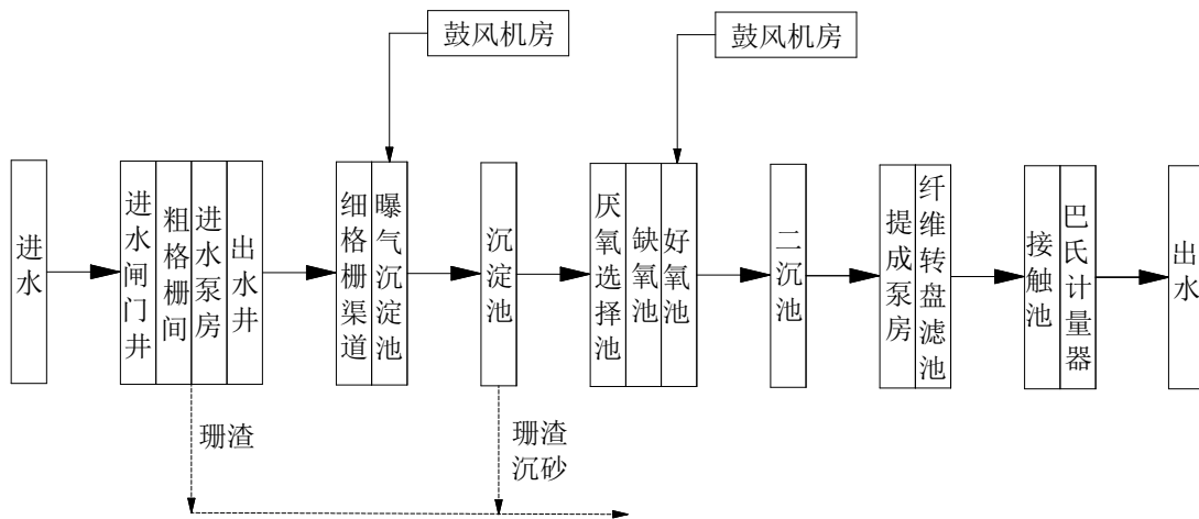
图 3 污水处理工艺流程图
