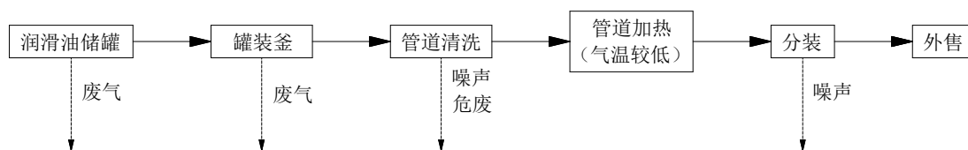
图1 生产工艺流程及产污环节图
