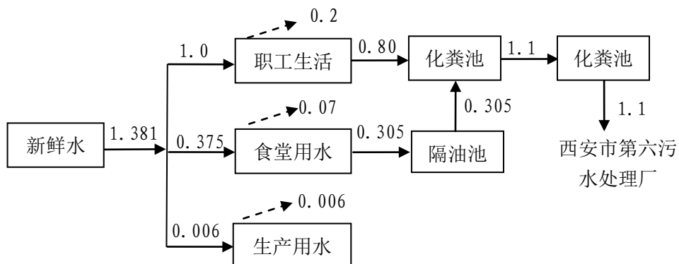
图 1 项目水量平衡图 (单位：m 3 /d)
