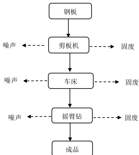
图2 机械加工工艺流程图
