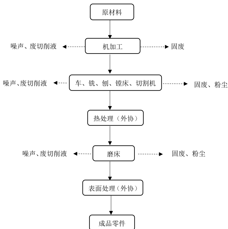
图2 机械零部件加工工艺流程图
