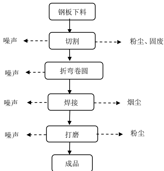
图 2 异形件加工工艺流程图
