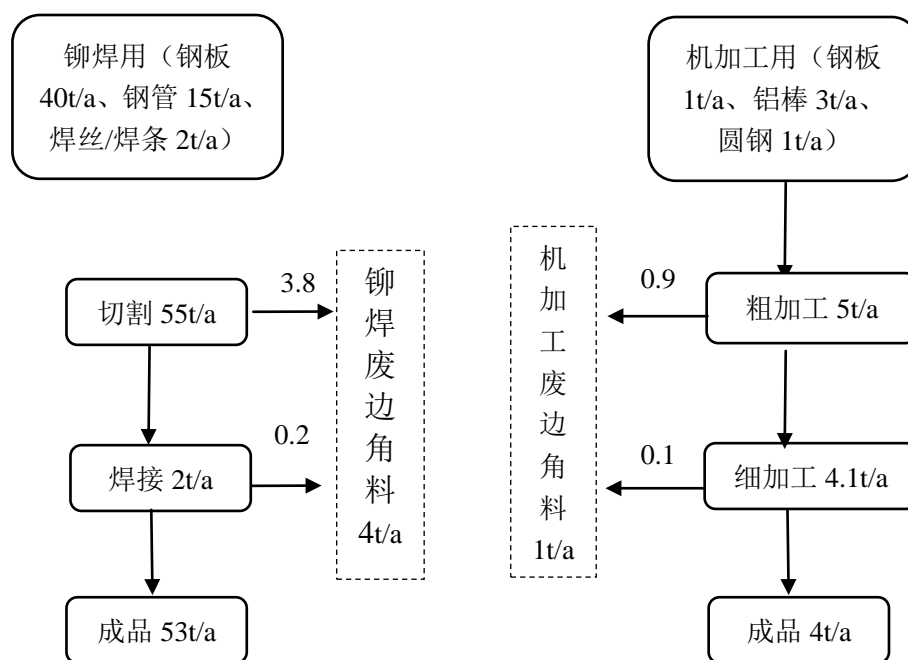
图 4 项目物料平衡图 (单位: t/a)
