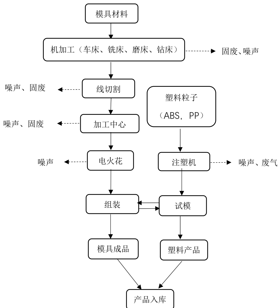
图2 模具加工工艺及各环节排污流程图
