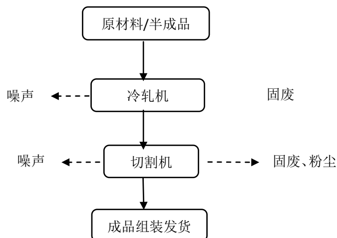
图3 卷闸门加工工艺流程图
