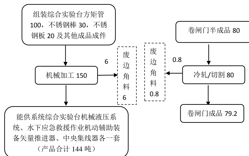
图 4 项目物料平衡图（单位：t/a）
