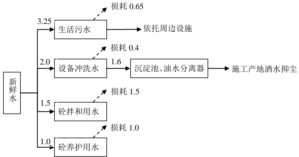
图 6 施工期水平衡图 单位：m 3 /d
