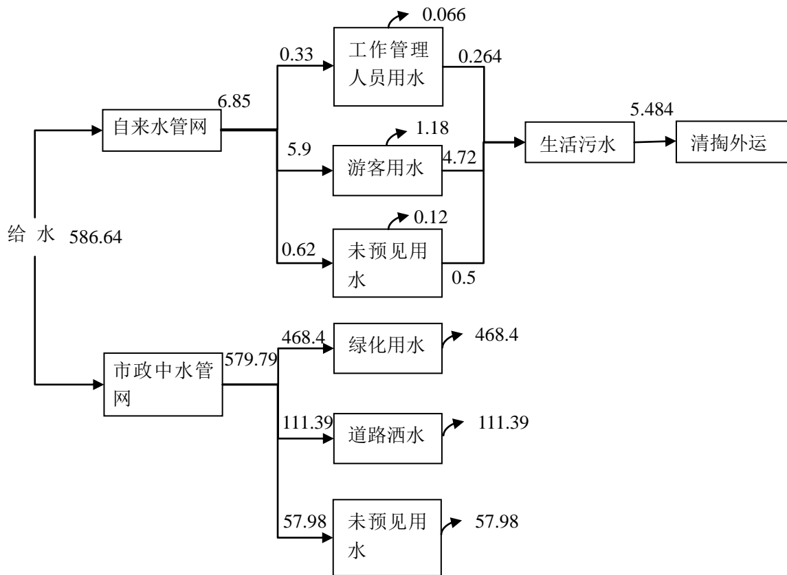
图 1 项目水平衡图(t/d)
