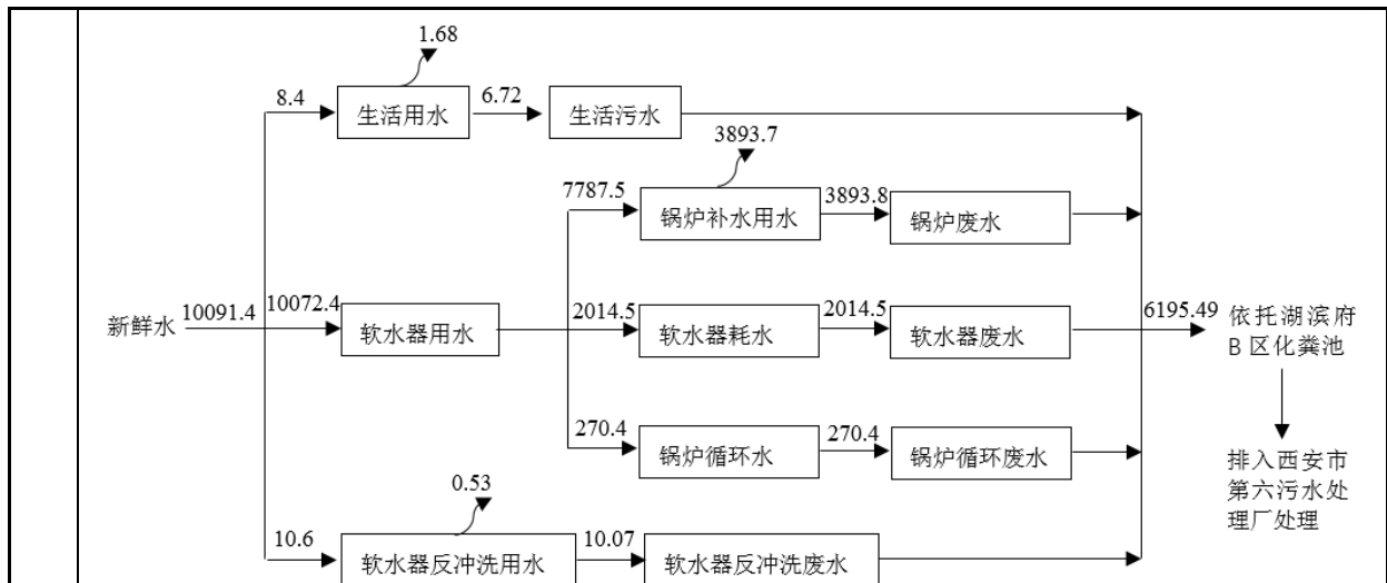
图 2-1 项目水平衡图 (m 3 /a)
