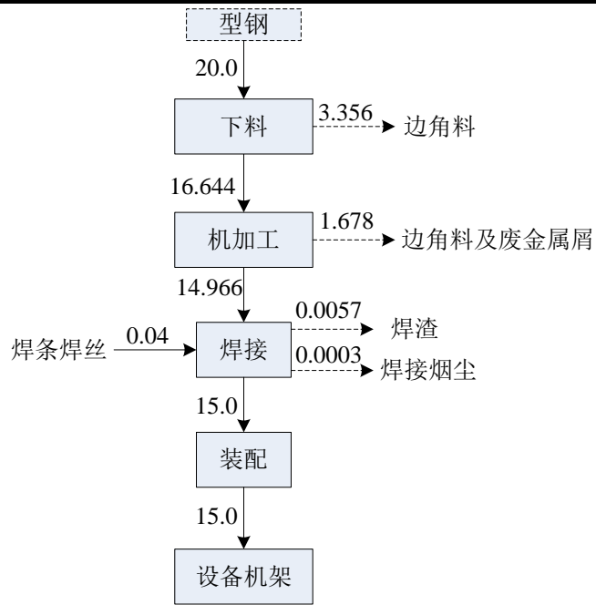
图 5 设备机架物料平衡图
