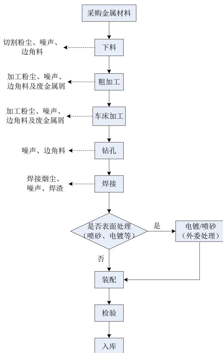
图 2 设备机架及金属零部件生产工艺流程及产污环节图
