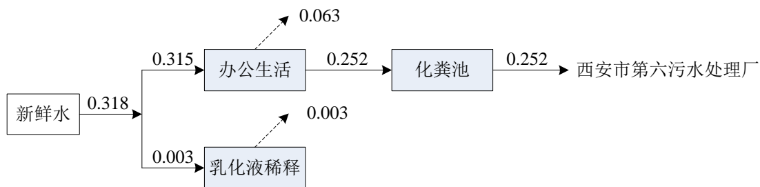
图1 项目水平衡图 单位: \text{m}^3/\text{d}
