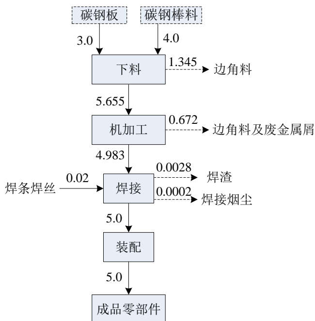
图 4 金属零部件物料平衡图
