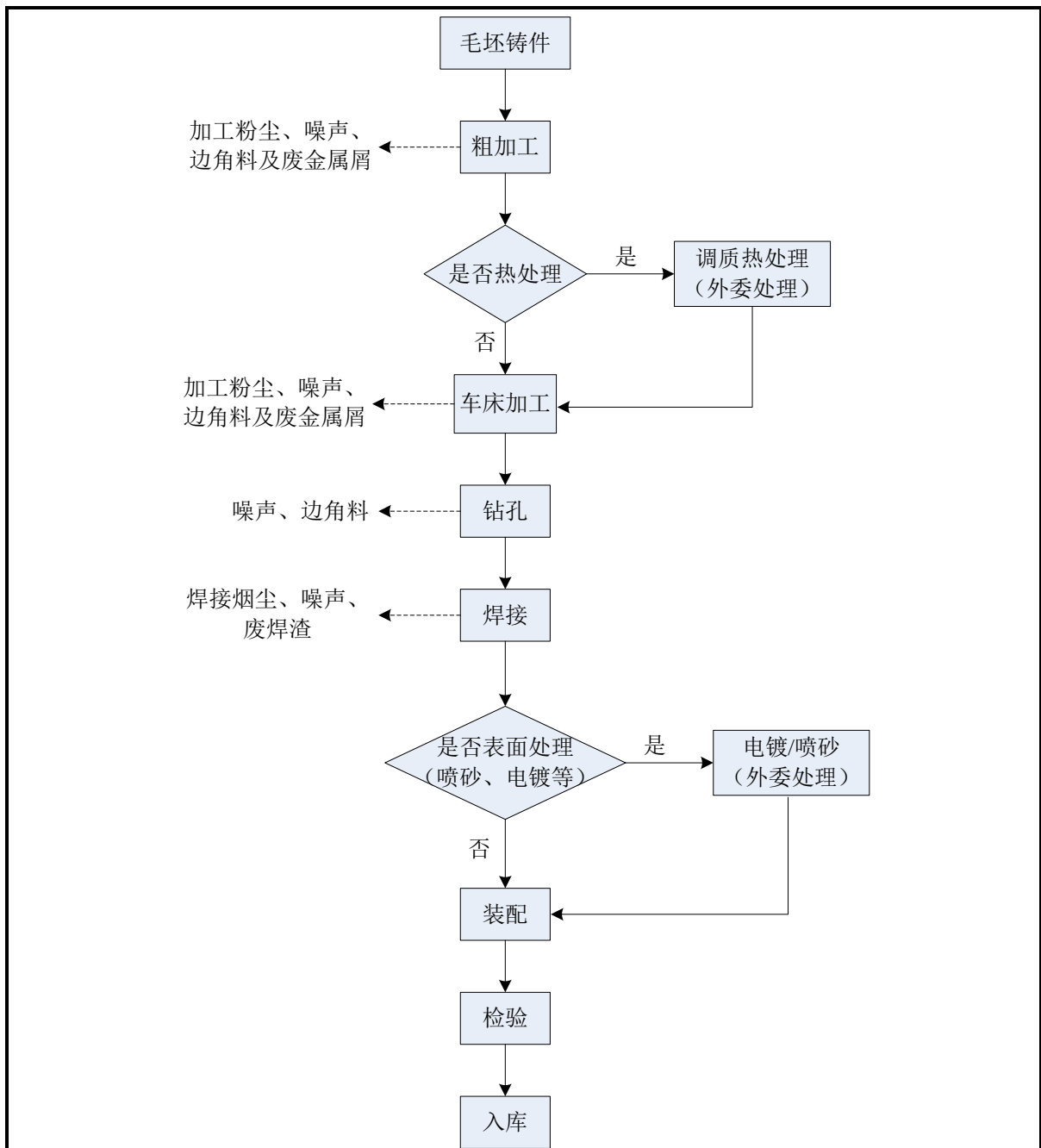
图3 非标设备生产工艺流程及产污环节图
