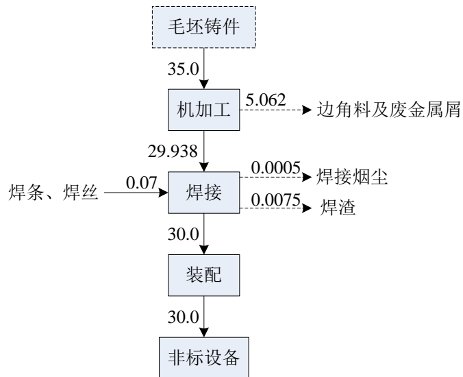
图 6 非标设备物料平衡图
