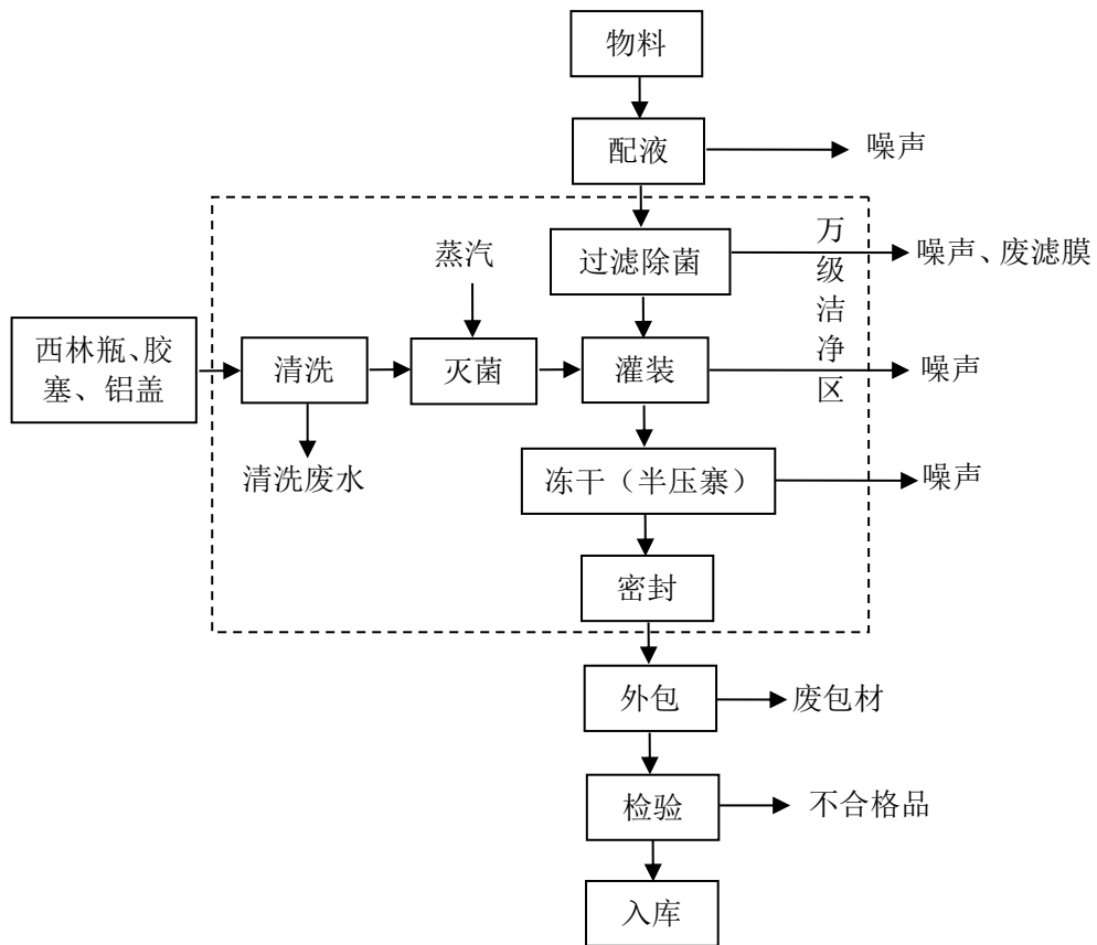
图 2-2 注射填充材料生产工艺流程
