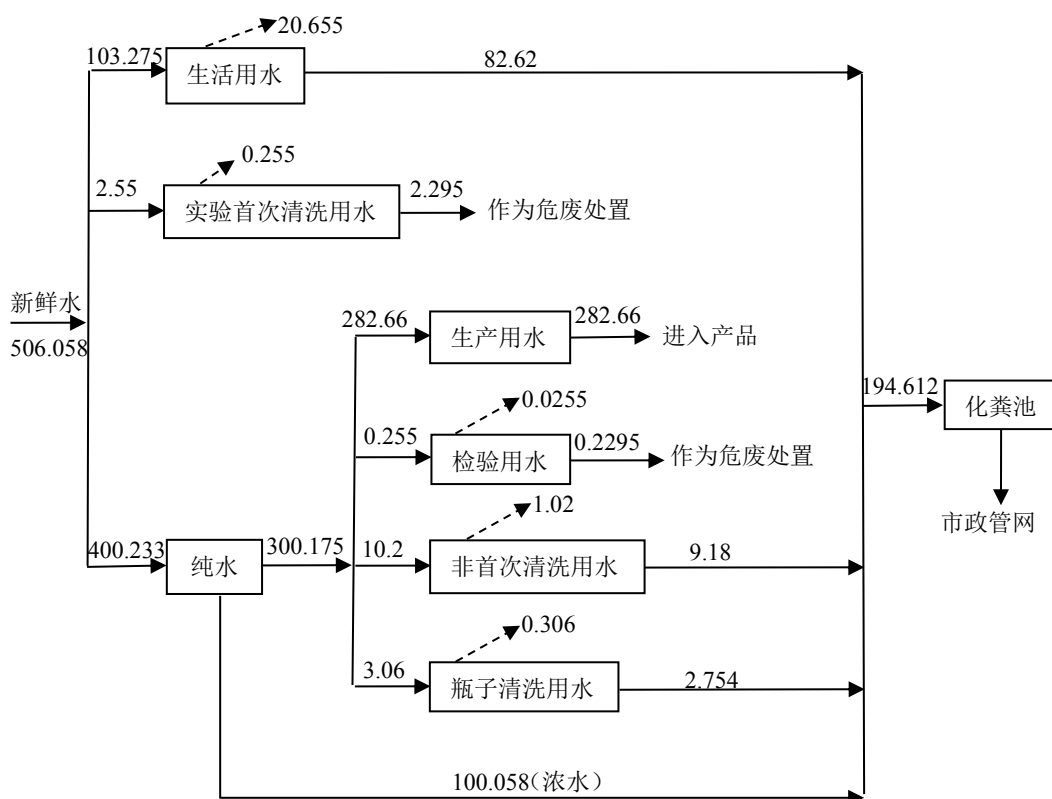
图 2-1 本项目用水平衡图 单位 m 3 /a
