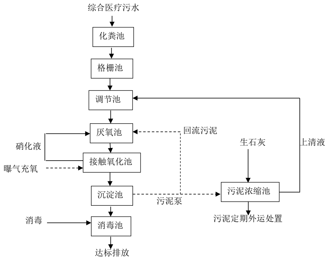
图5 医院废水处理站工艺流程
