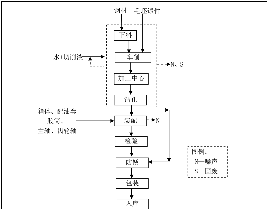
图 3 采煤设备配件代加工及组装生产工艺及产污节点图
