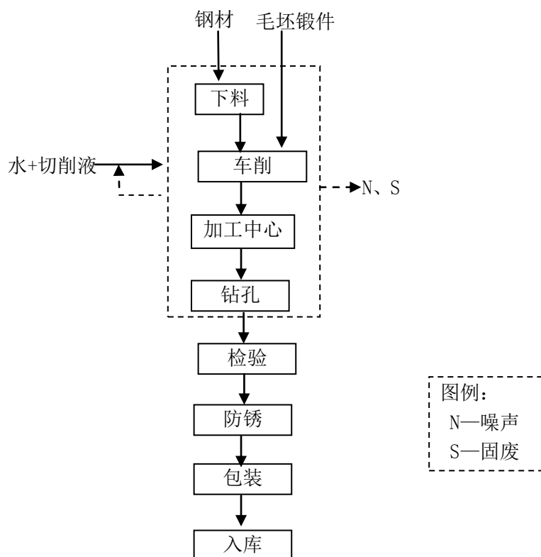
图2 减速器配件机械加工生产工艺及产污节点图
